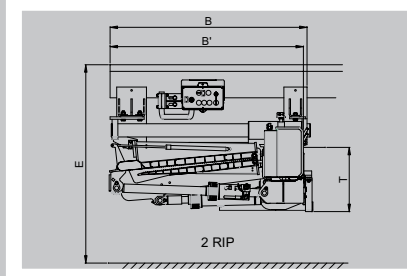
Vista lateral de la trampa elevadora montada - Plano de 2 dobleces
