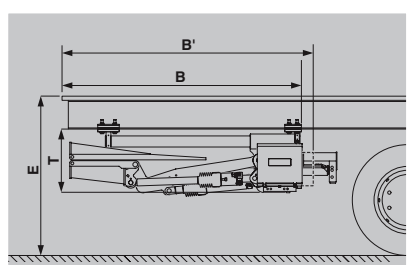
Montaje rápido para semirremolque - Plato 1 plegado
